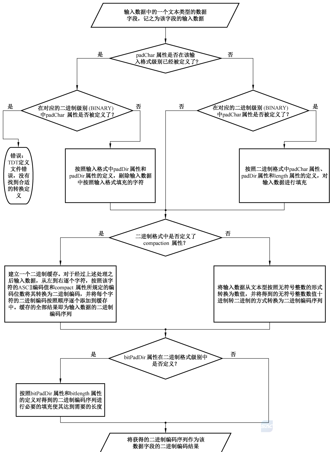
图 8 编码过程填充流程
