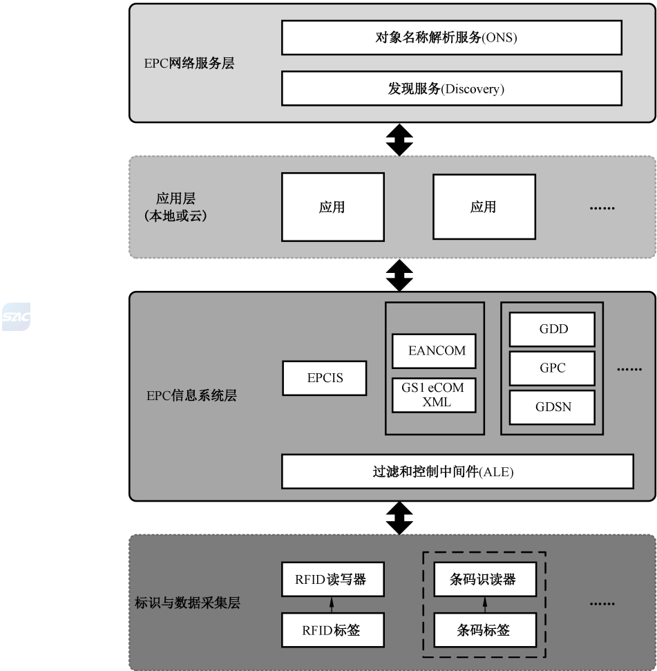
图 1 EPC 系统架构图
