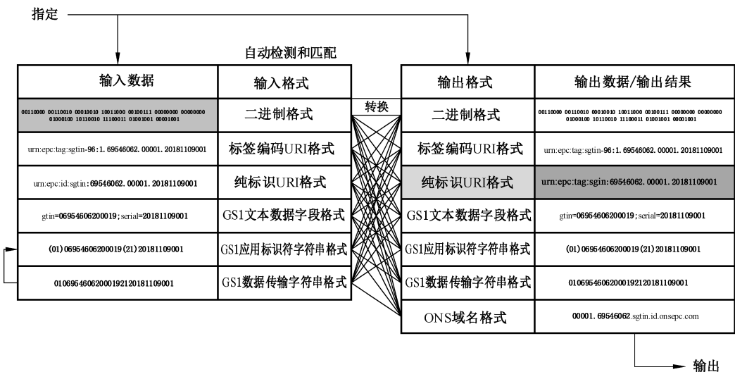
图 3 标签数据转换过程的输入与输出
