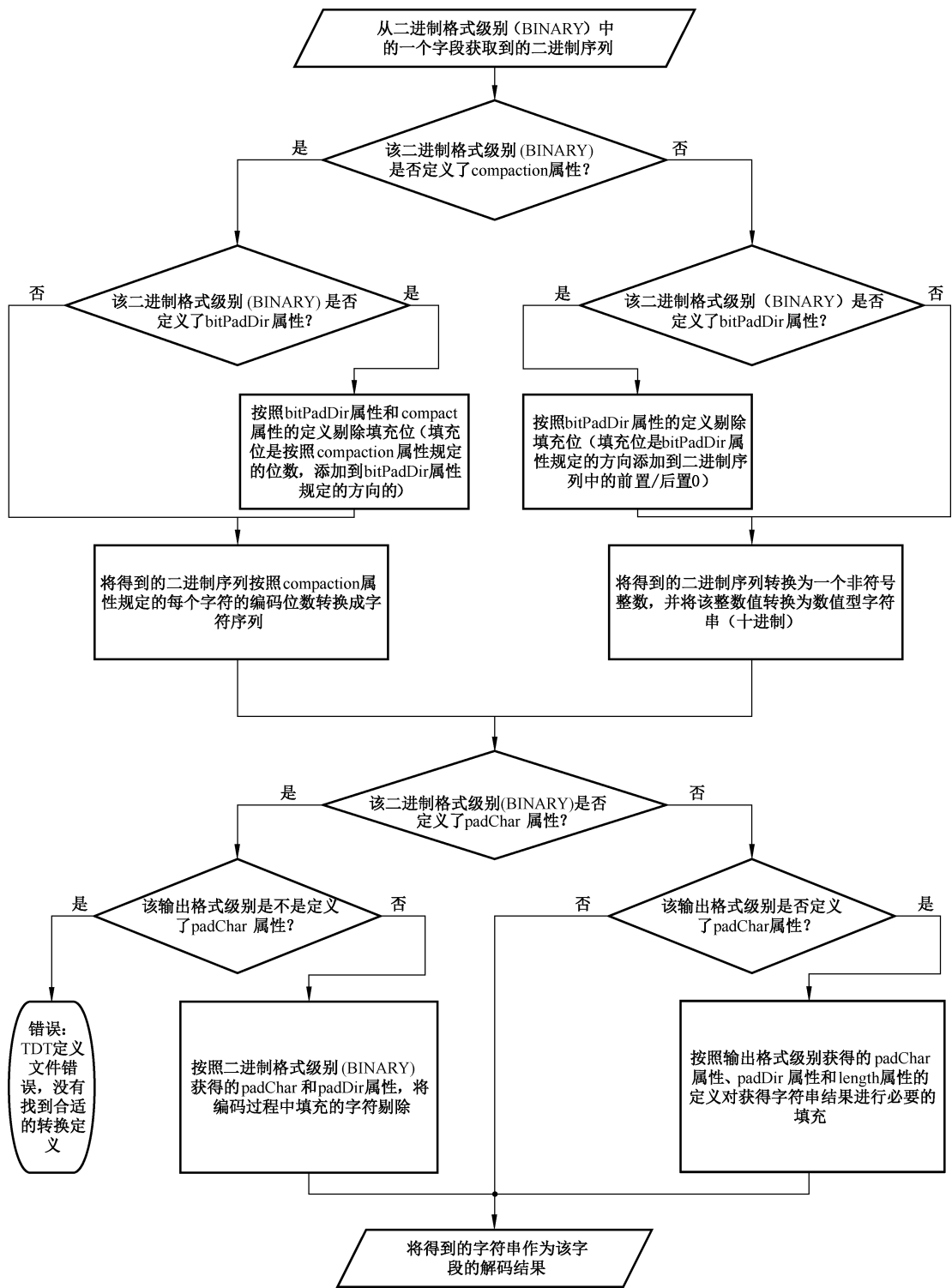
图 9 解码过程填充流程
